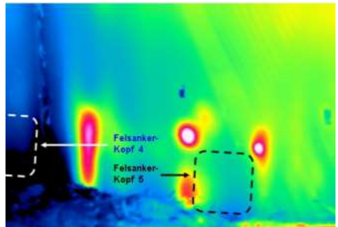
5. Felsanker-Kopf in der Fläche 4. Felsanker-Kopf hinter der Vorschubbahn
